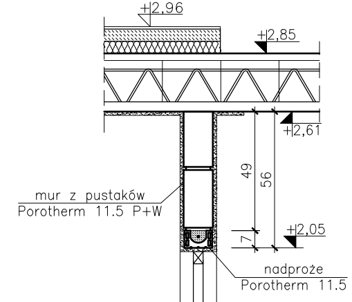
Nadproże wewnętrzne ściana działowa
