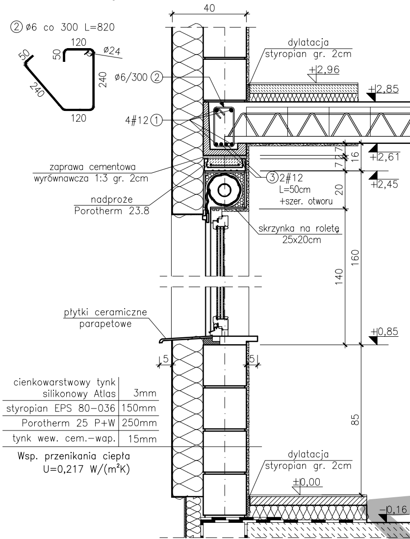
Nadproże w ścianie zewnętrznej część mieszkalna - parter
