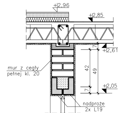
Alternatywnie - nadproża L19
