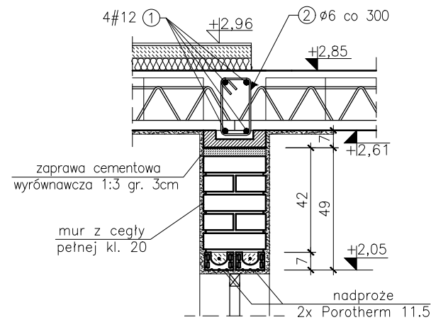
Nadproże wewnętrzne ściana konstrukcyjna
