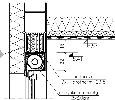
Nadproże wewnętrzne ściana konstrukcyjna
