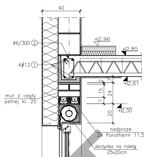
Nadproże w ścianie zewnętrznej w garażu, kotłowni
